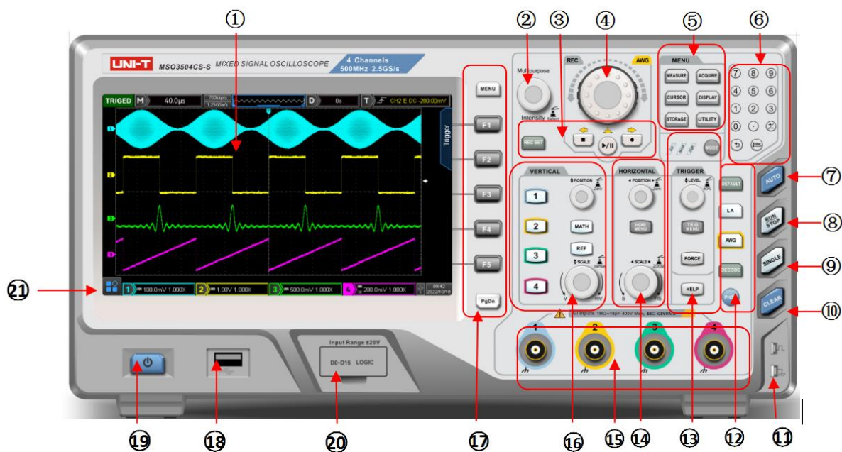
图 3 示波器前面板
